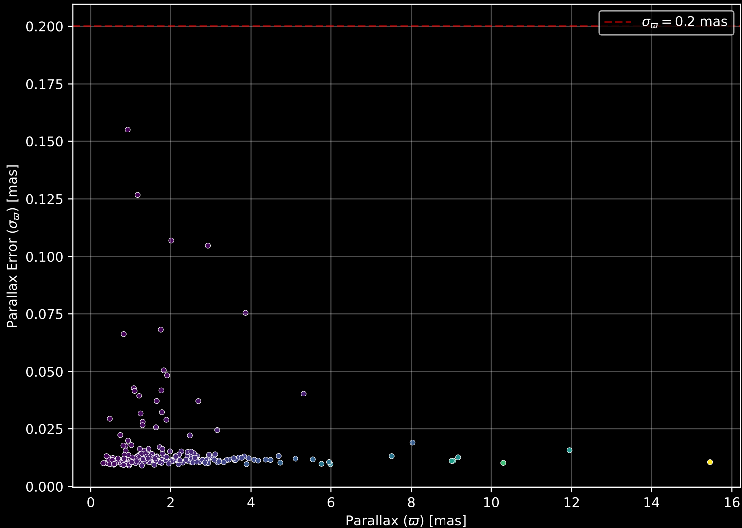
GALAH DR4 Field: [7147] Parallax Quality (n= 215)
