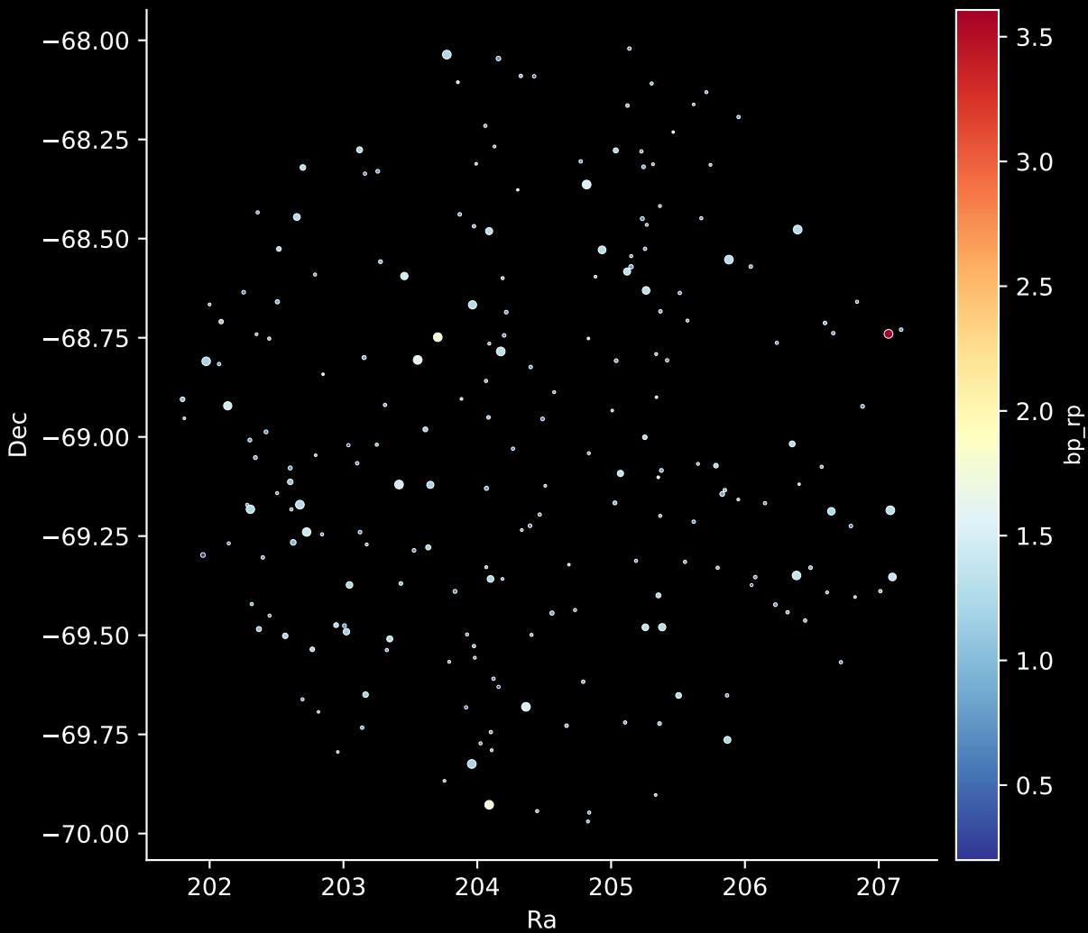
GALAH DR4 Field: [7147] Stars: 215
