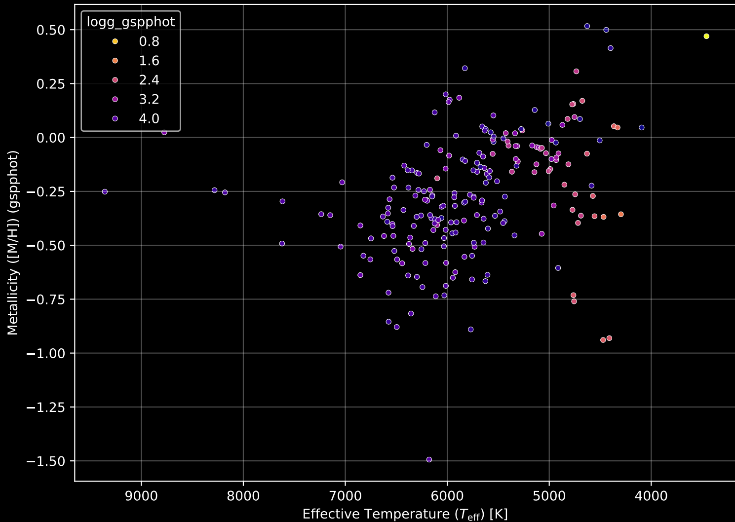
GALAH DR4 Field: [7147] Stellar Population Parameters (n= 215)
