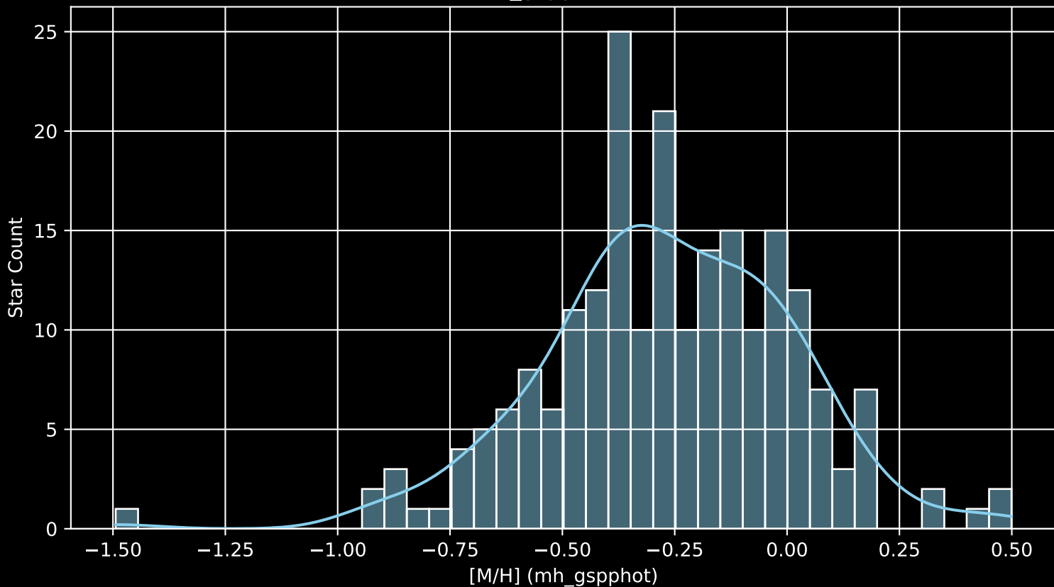
GALAH DR4 Field: [7147] [M/H] (mh_gspphot) (n= 214)
